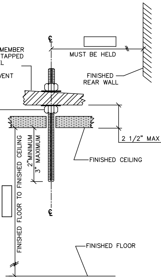
SECTION A-A
