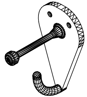
COMBINATION COAT HOOK / DOOR STOP
